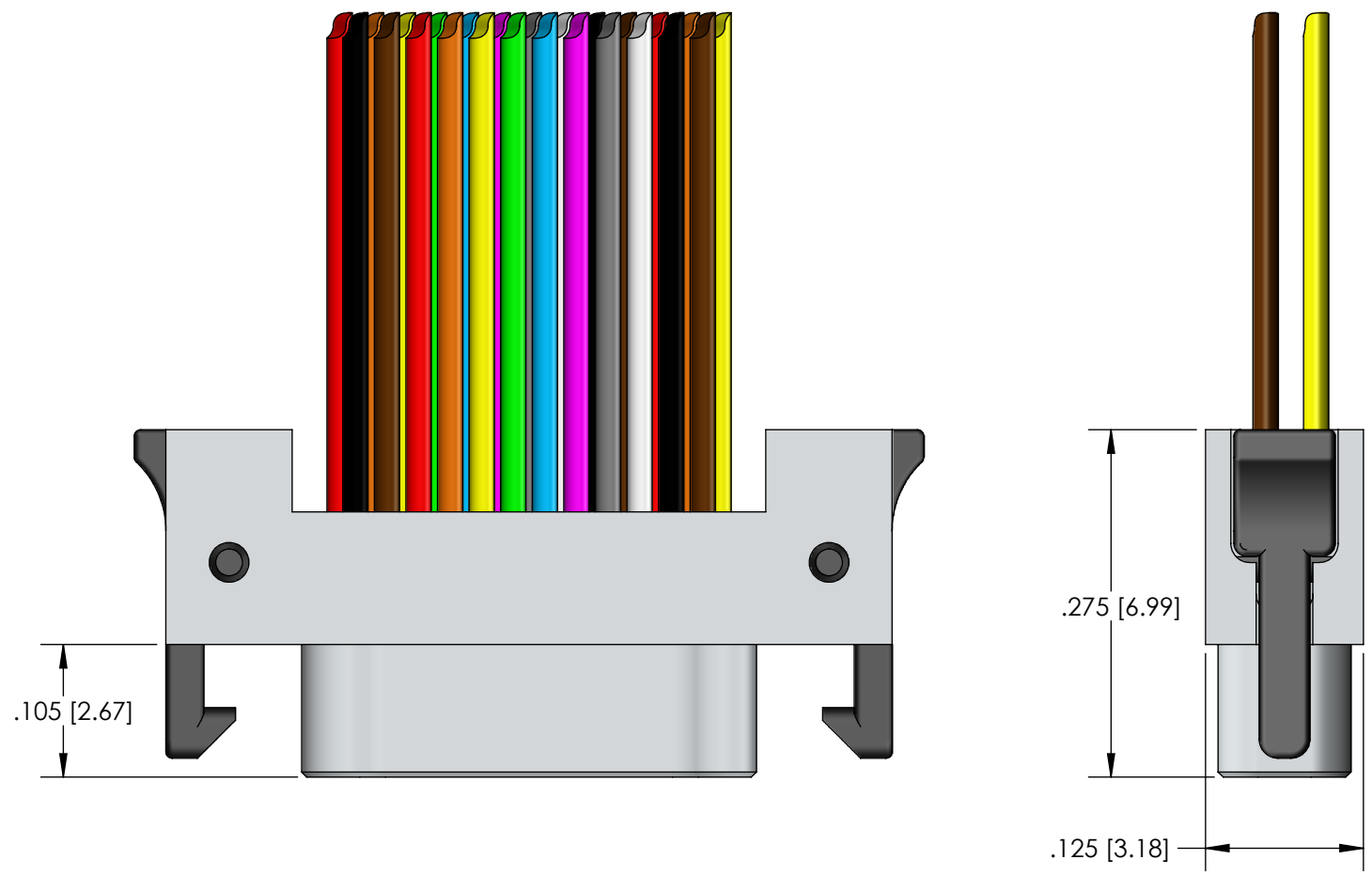
PLUG (PINS)
