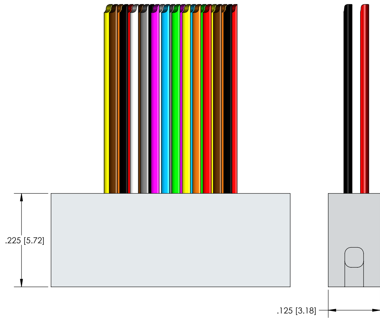
RECEPTACLE (SOCKETS)
