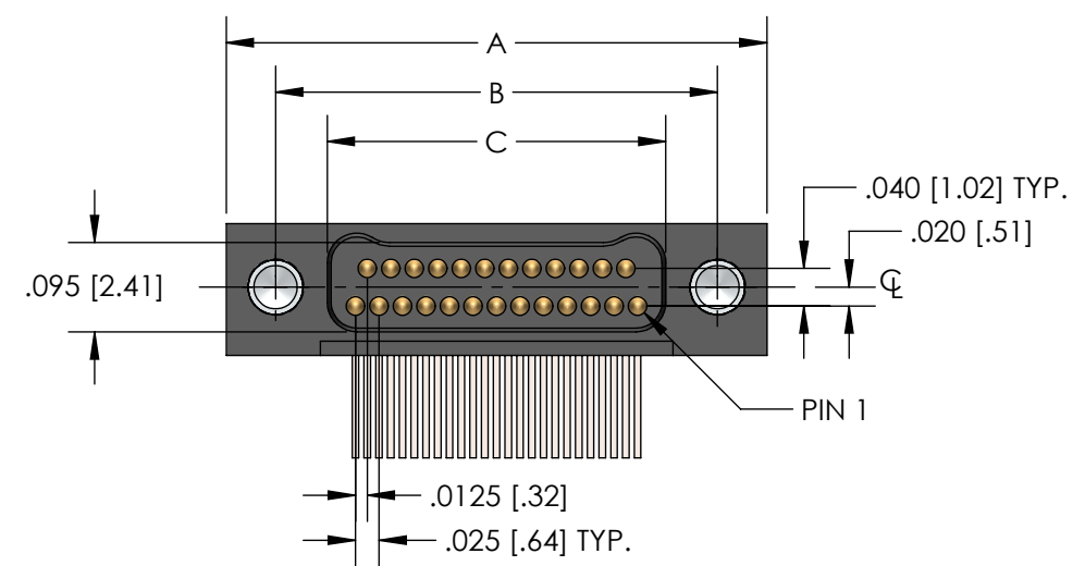
PLUG (PINS)
