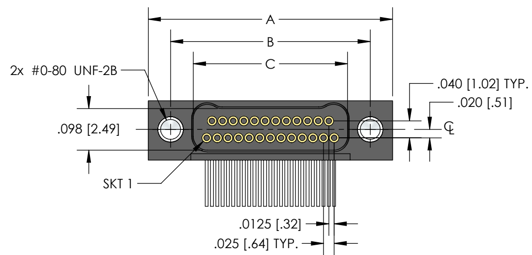
RECEPTACLE (SOCKETS)
